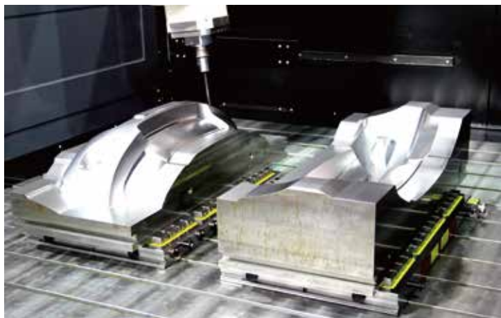
5軸加工機で金型を永電磁チャックで固定して機械加工
