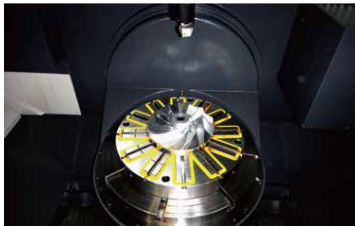
5軸加工機でインペラーを機械加工
